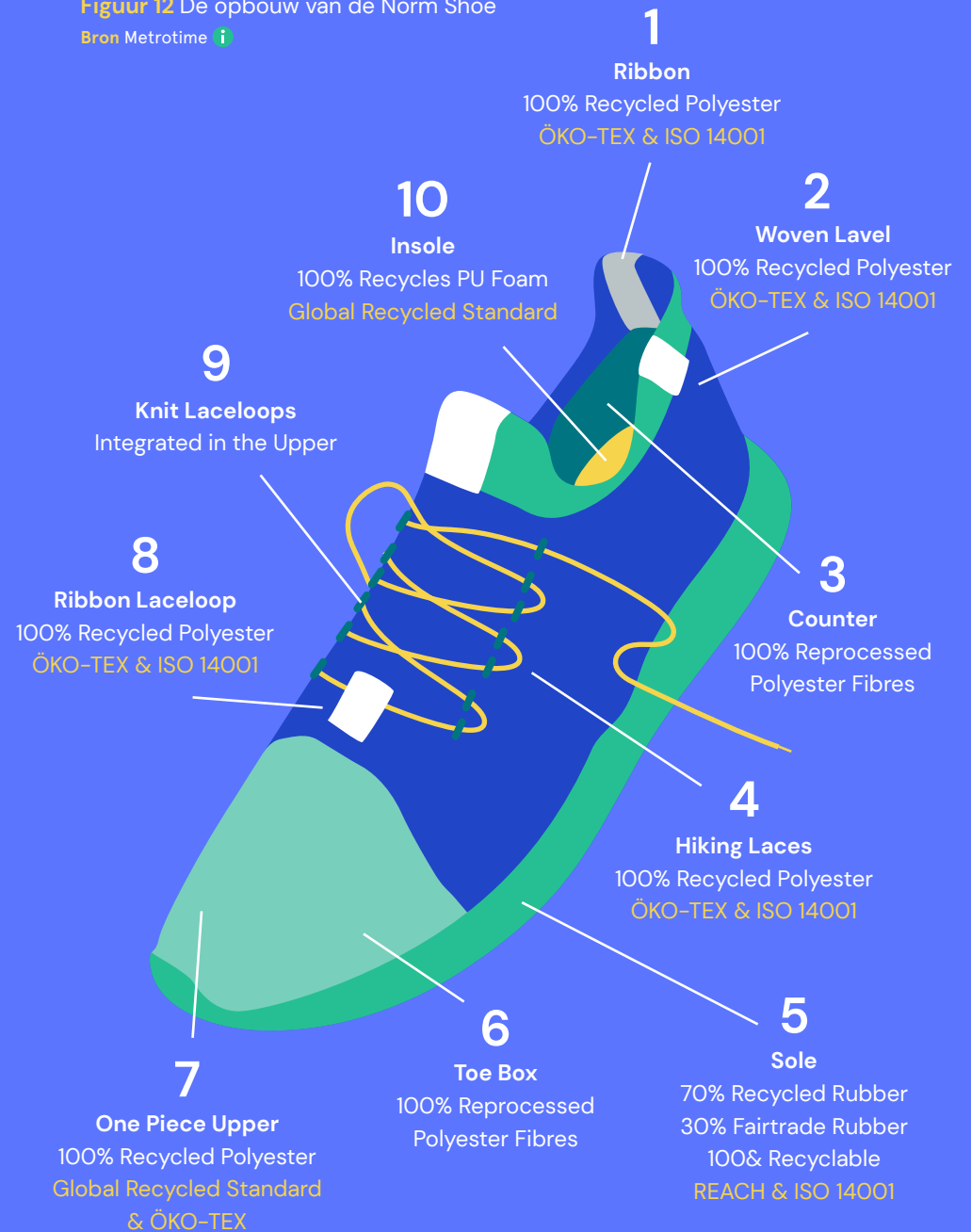
Figuur 12 De opbouw van de Norm Shoe
